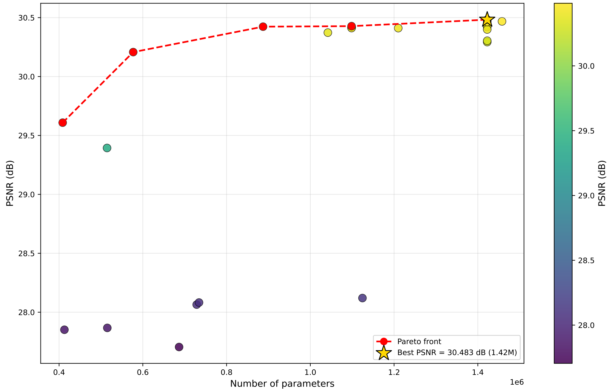
PSNR vs #Parameters — SwinT
